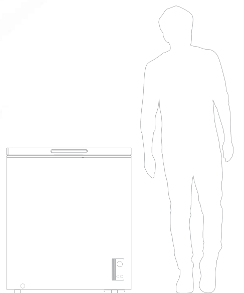
Dimensiones (ancho x fondo x alto) 112,5 x 61 x 83,5 cm.
